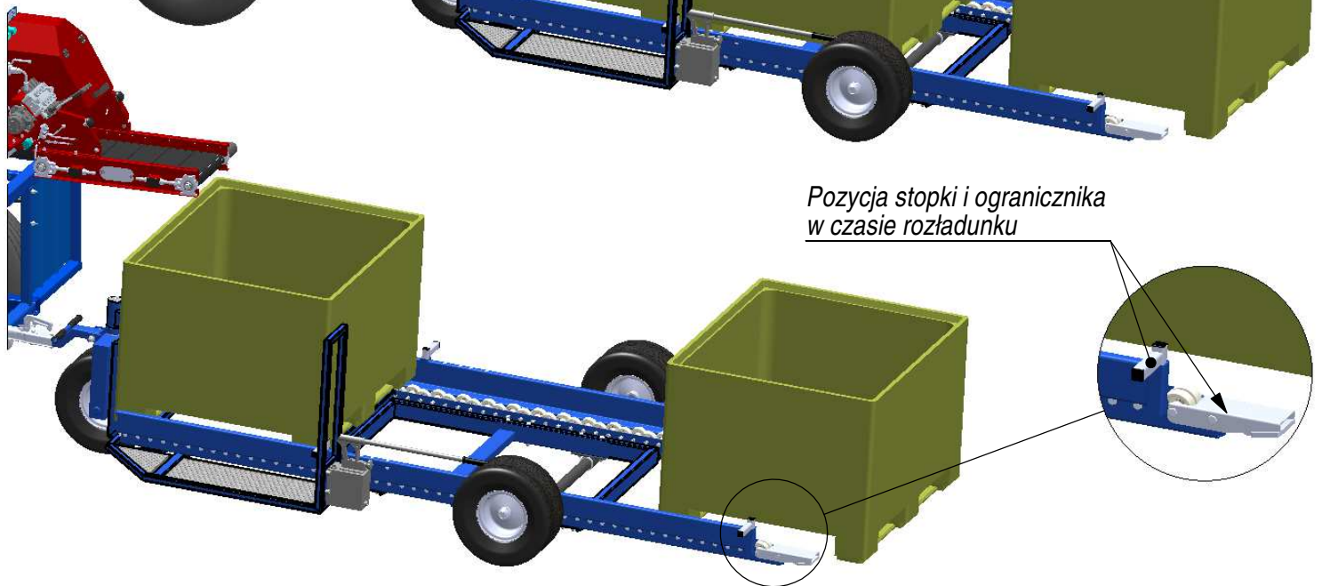
Kombajn Jarek 5 Opcja: z wózkiem samowyładowczym na 3 skrzyniopalety Widok: rozładunek skrzyniopalet
