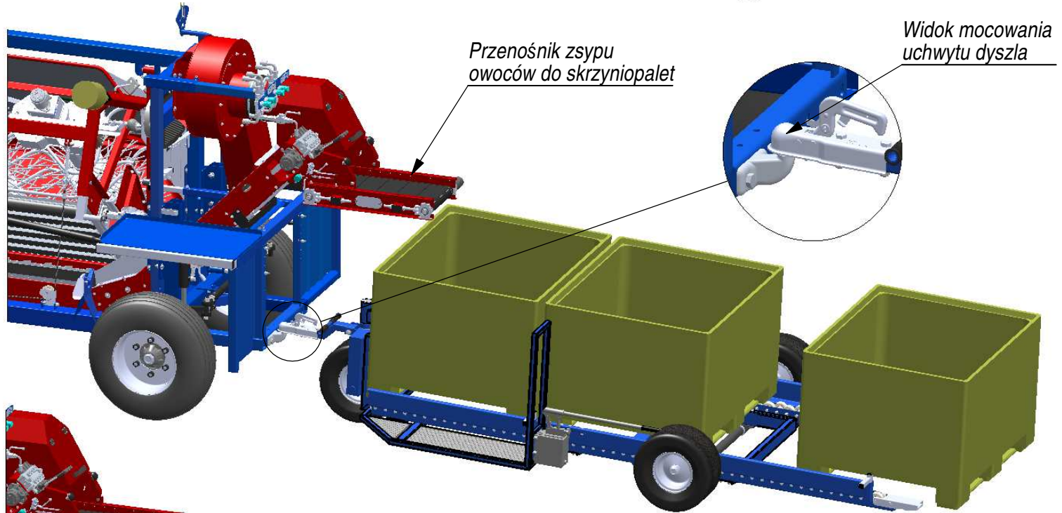
Kombajn Jarek 5 Opcja: z wózkiem samowyładowczym na 3 skrzyniopalety Widok: zbiór do skrzyniopalet
